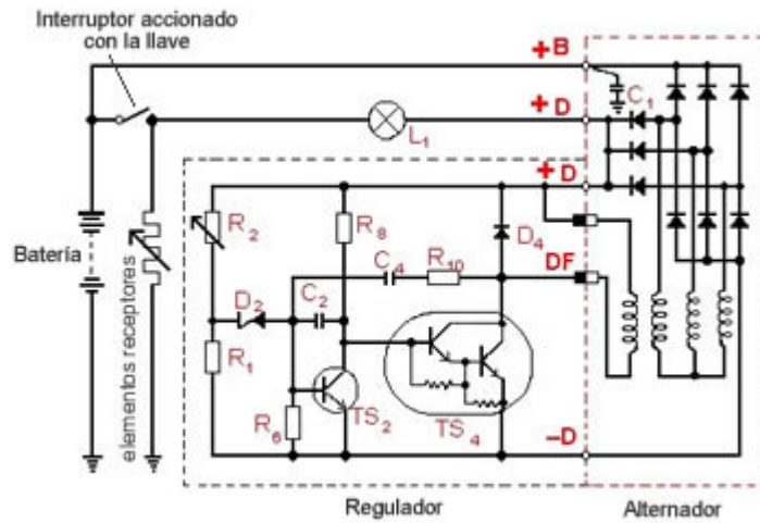
Esquema eléctrico de un alternador con su regulador electrónico mas el circuito de carga que lo rodea formado por la batería, la lampara de control, el interruptor de la llave y los circuitos de los elementos receptores (luces, encendido, elevallas etc.).
